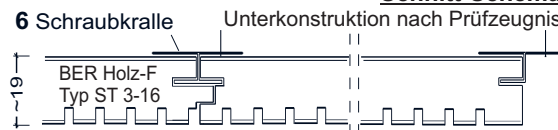
Schnitt-Schema
