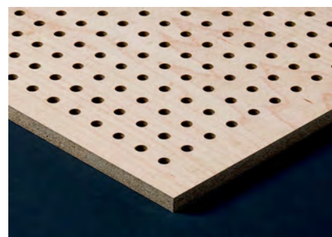
BER Holz-F A-BG Akustikplatte Typ L 6/12-16
