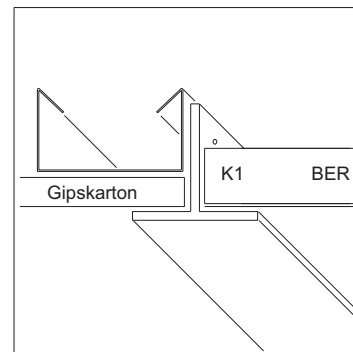
T-Profil 40/40/3
