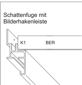
Wandprofil 501
